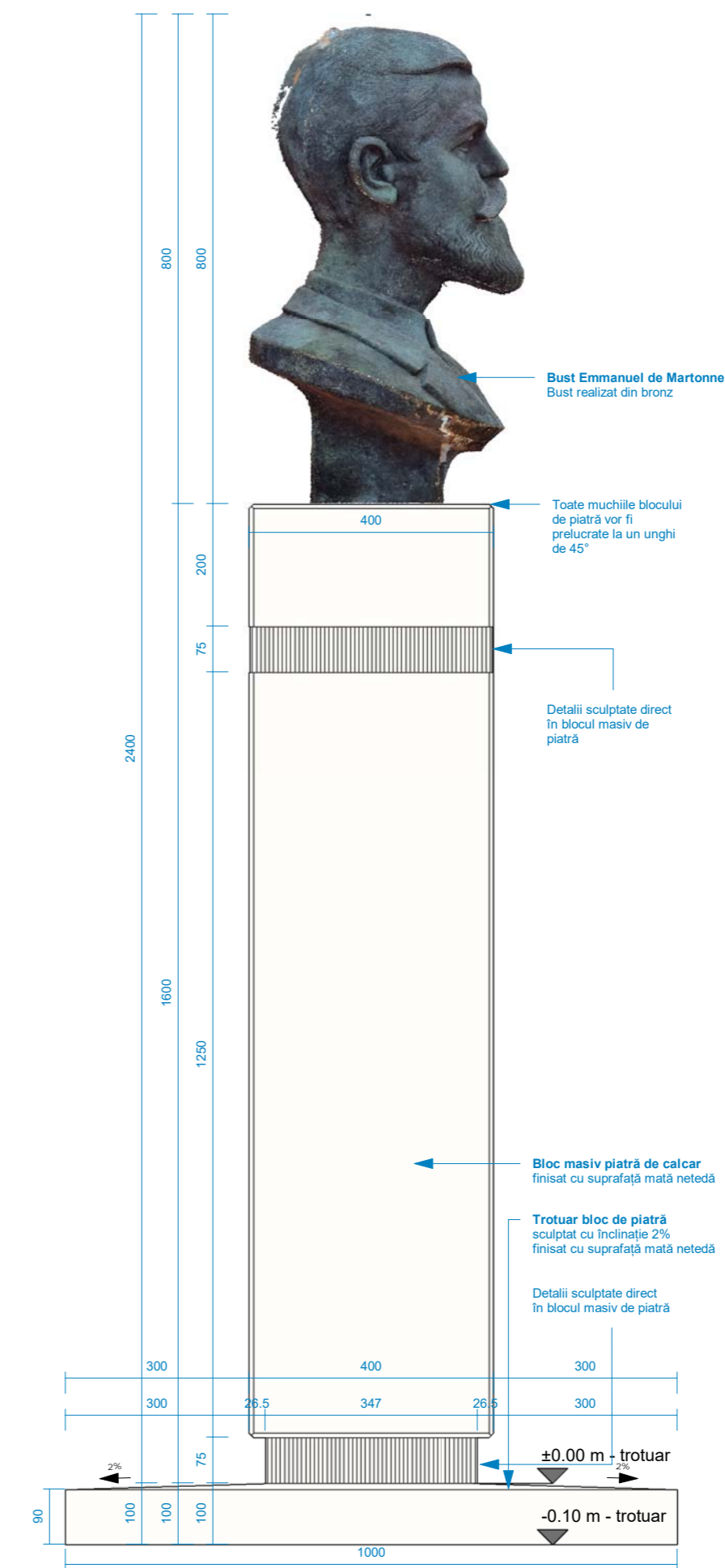
Elevație laterală stânga sc: 1:10
