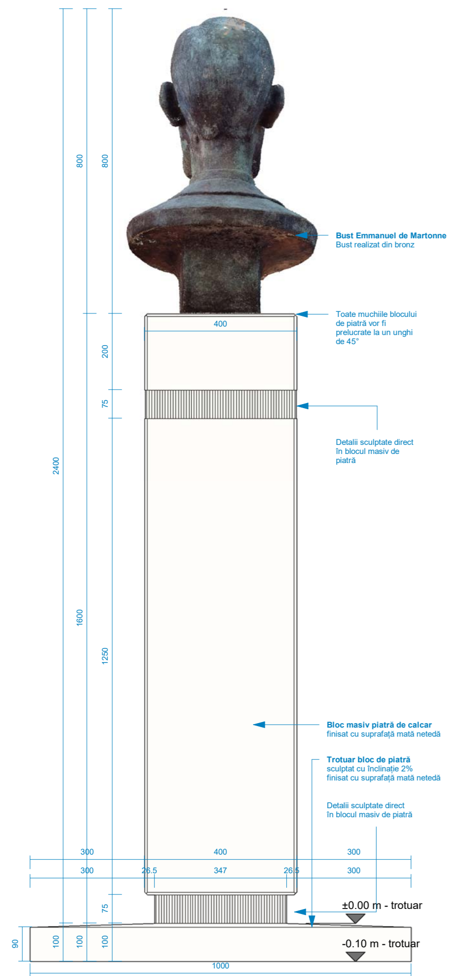
Elevație posterioară sc: 1:10
