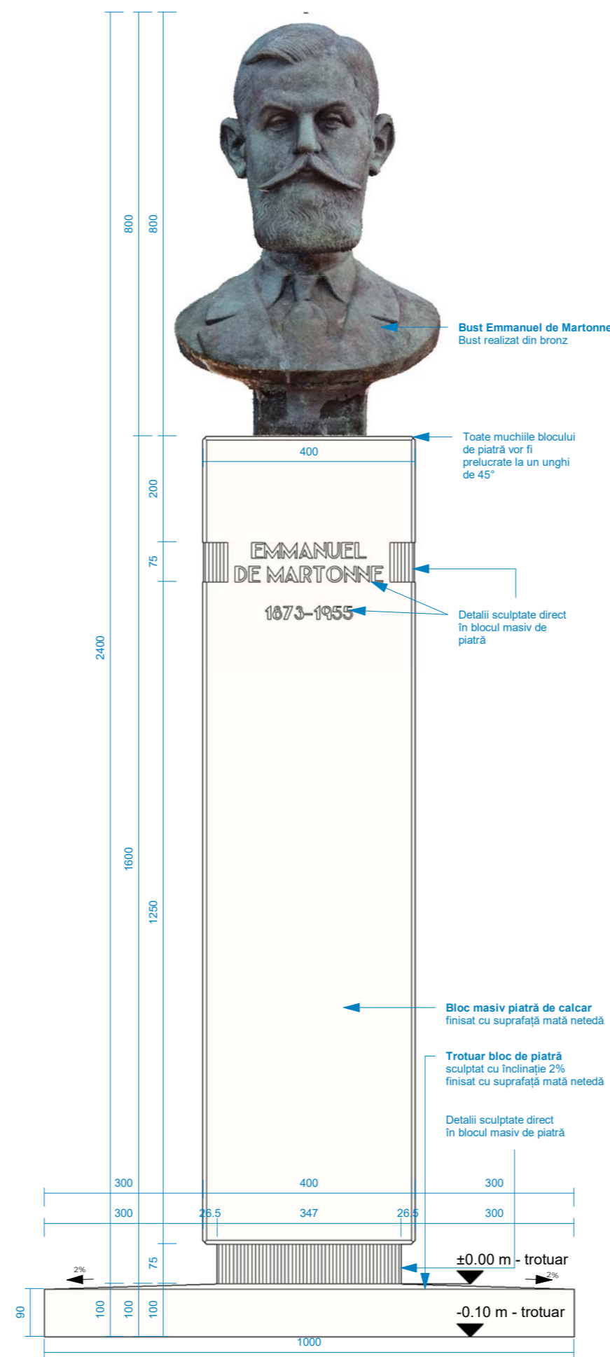
Elevație frontală sc: 1:10
