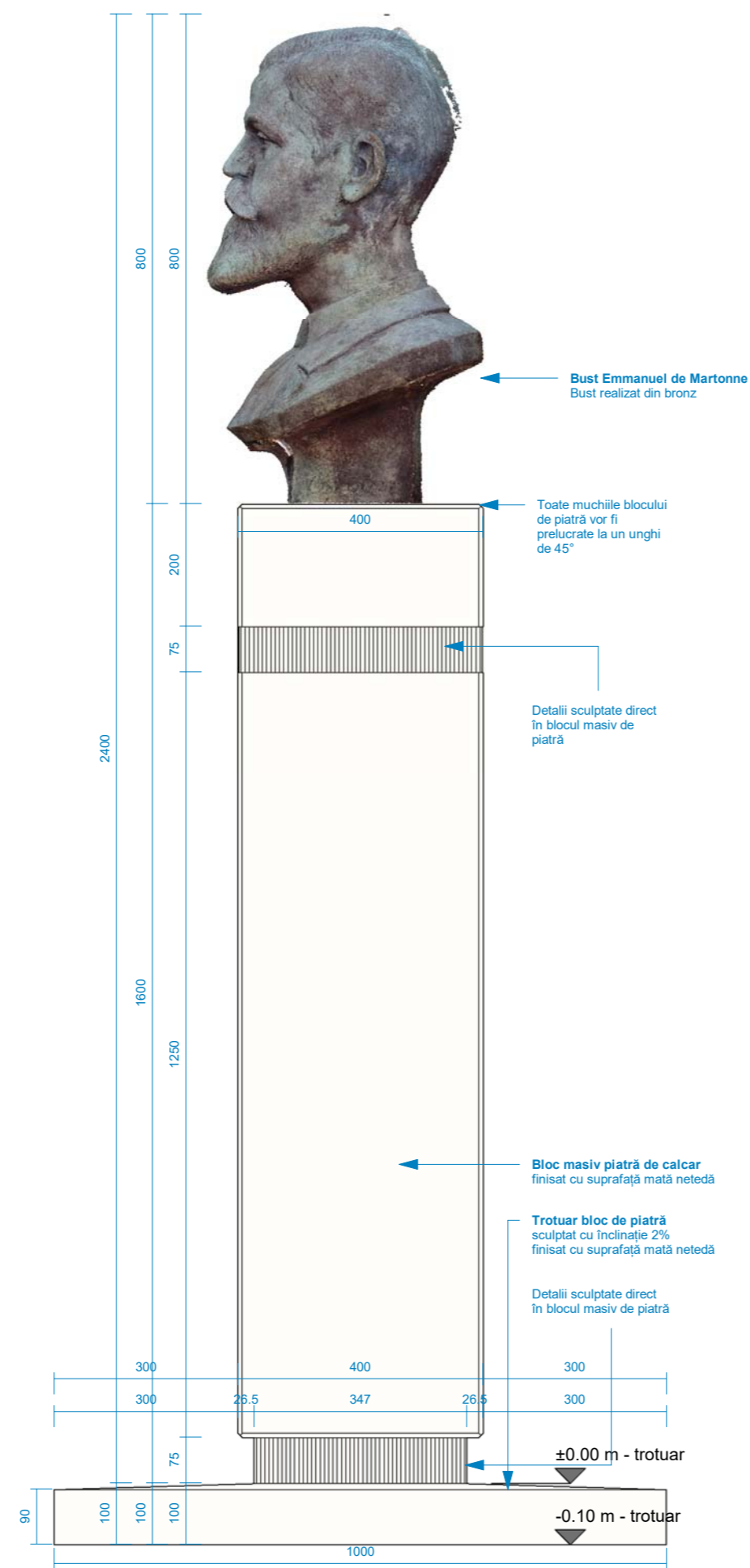
Elevație laterală dreapta sc: 1:10
